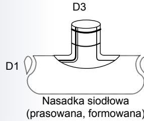
Nasadka siodłowa (formowana)
