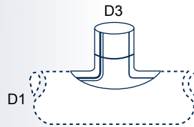
Sattelstutzen (gepresst, handgebaut)
